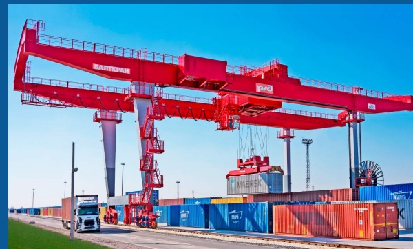
КОНТЕЙНЕРНЫЙ КРАН RMG Г/П 45 Т, ТЛЦ «ВОСТОК-ЗАПАД», ЧЕРНЯХОВСК, РОССИЯ.
